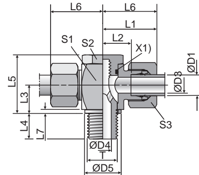
X1) O-ring OR
